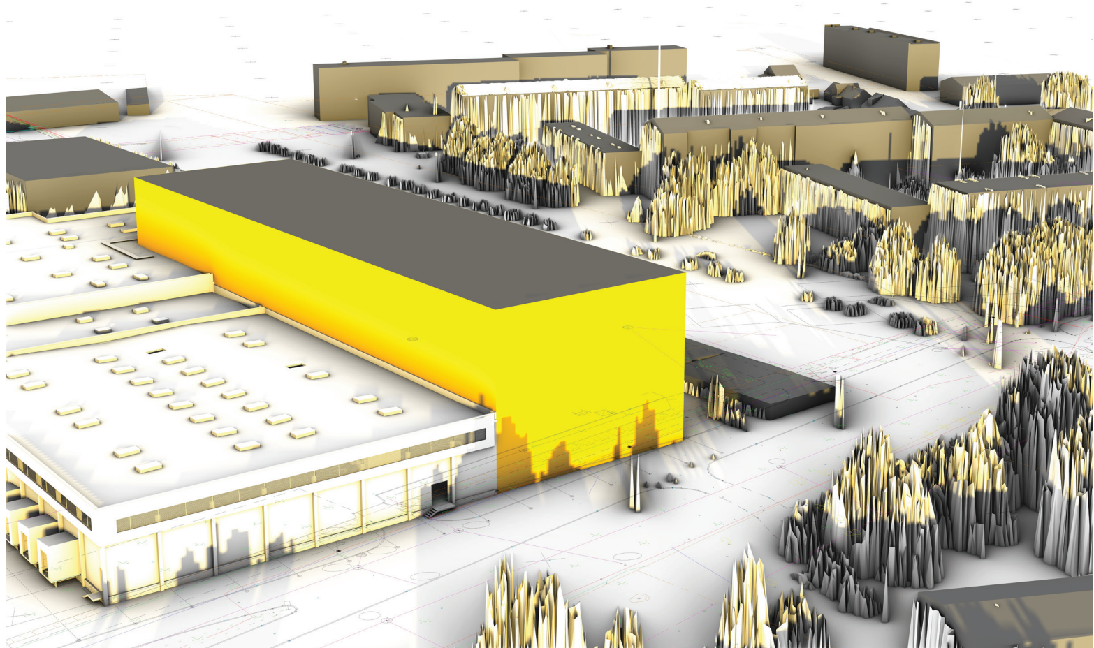
23 m kõrguse hoonemahu vari 21. detsember, kell 13.00
