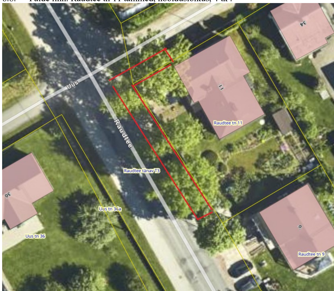
6.8. Paide linn. Raudtee tn 11 tammed, hoolduslõikus, 4 tk .
